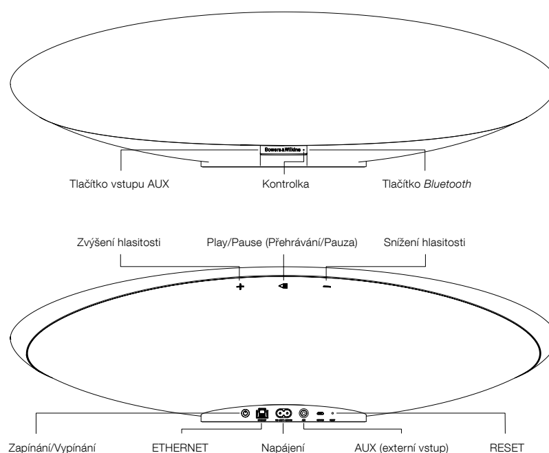
Obrázek 1 Ovládací prvky a terminály
